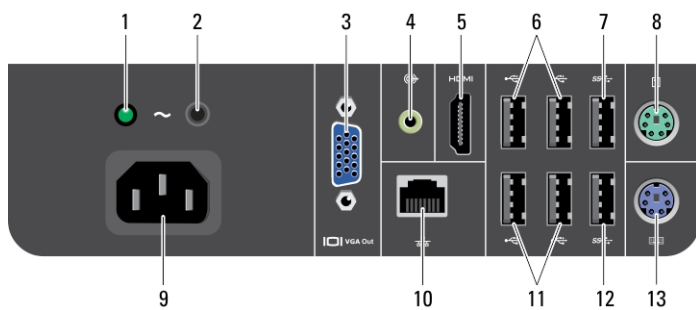
图 3: 背面板视图
