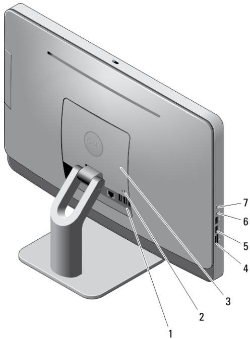
图 2: 背面视图
